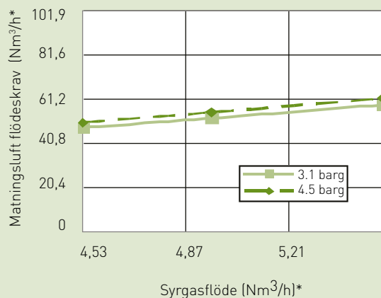
Model AS-E syrgasgenerator matningsluftskrav** (93% nominell syrgas)
